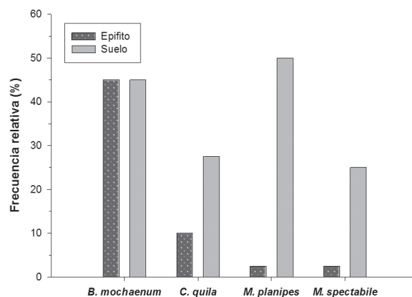
FIGURA 1. Abundancia (frecuencia relativa) de las especies presentes como epífitas accidentales, comparada con su abundancia en el suelo, en un bosque templado lluvioso del sur de Chile. / Abundance (relative frequency) of species that occur as accidental epiphytes, compared with their abundance on the ground, in a temperate rainforest in southern Chile.
